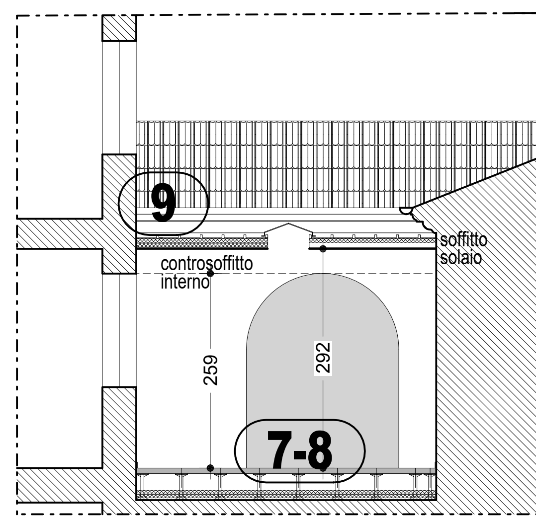
Sezione A-A
